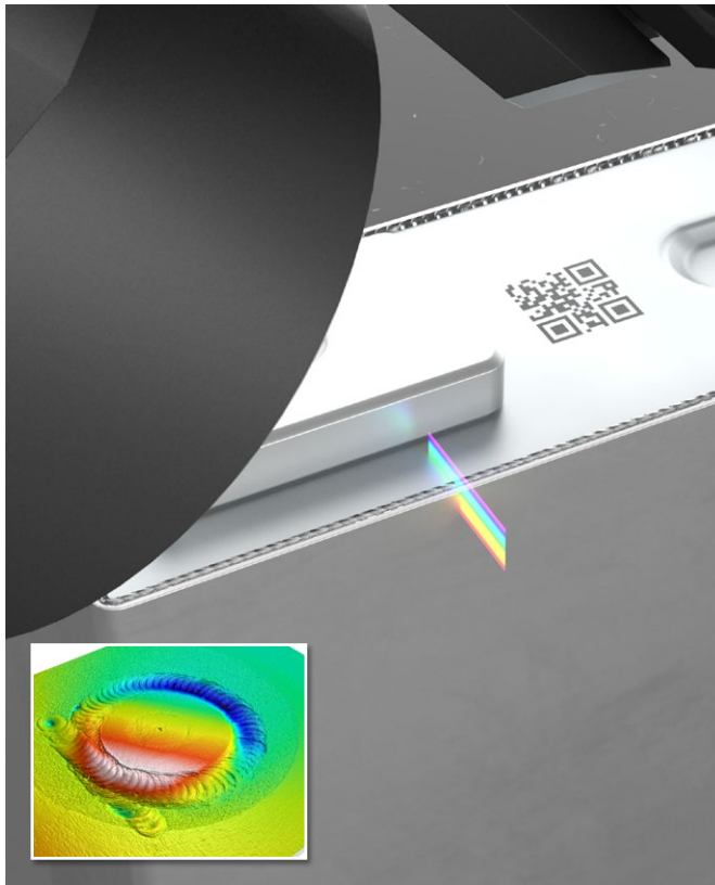
焊缝检测(极耳、注液口、汇流排模组)
