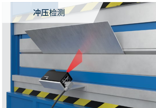
运用线激光轮廓传感器来确定折弯机的最终弯曲角度
