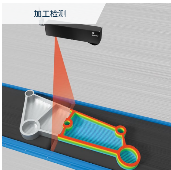
CNC成品扫描, 验证容差范围内的深度和孔尺寸
