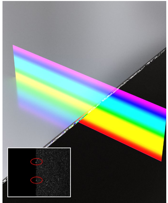
分切工艺中的毛刺检测
