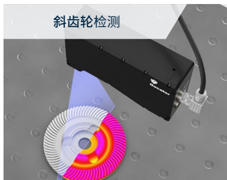
Gocator扫描复杂的金属物表面, 每个轮廓 4200个数据点
