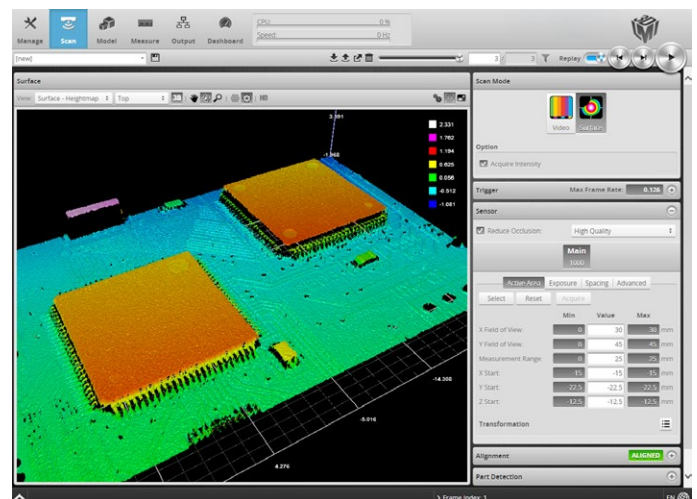
Gocator 基于浏览器的图形用户界面,上图展示电路板的三维扫描
